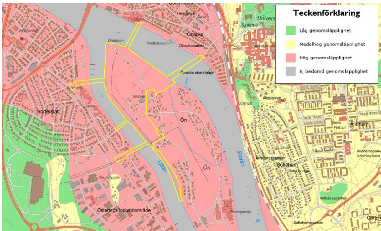
Figur 7. Genomsläpplighetskarta över planområdet (SGU, 2020).
