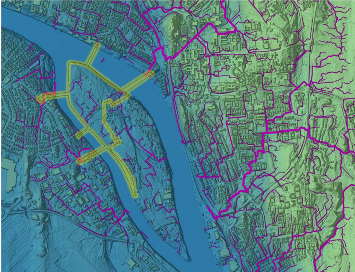
Figur 10. Flödeslinjer för avrinningen inom planområdet (ScalگوLive, 2020). Flödets storlek representeras av linjetjockleken.
