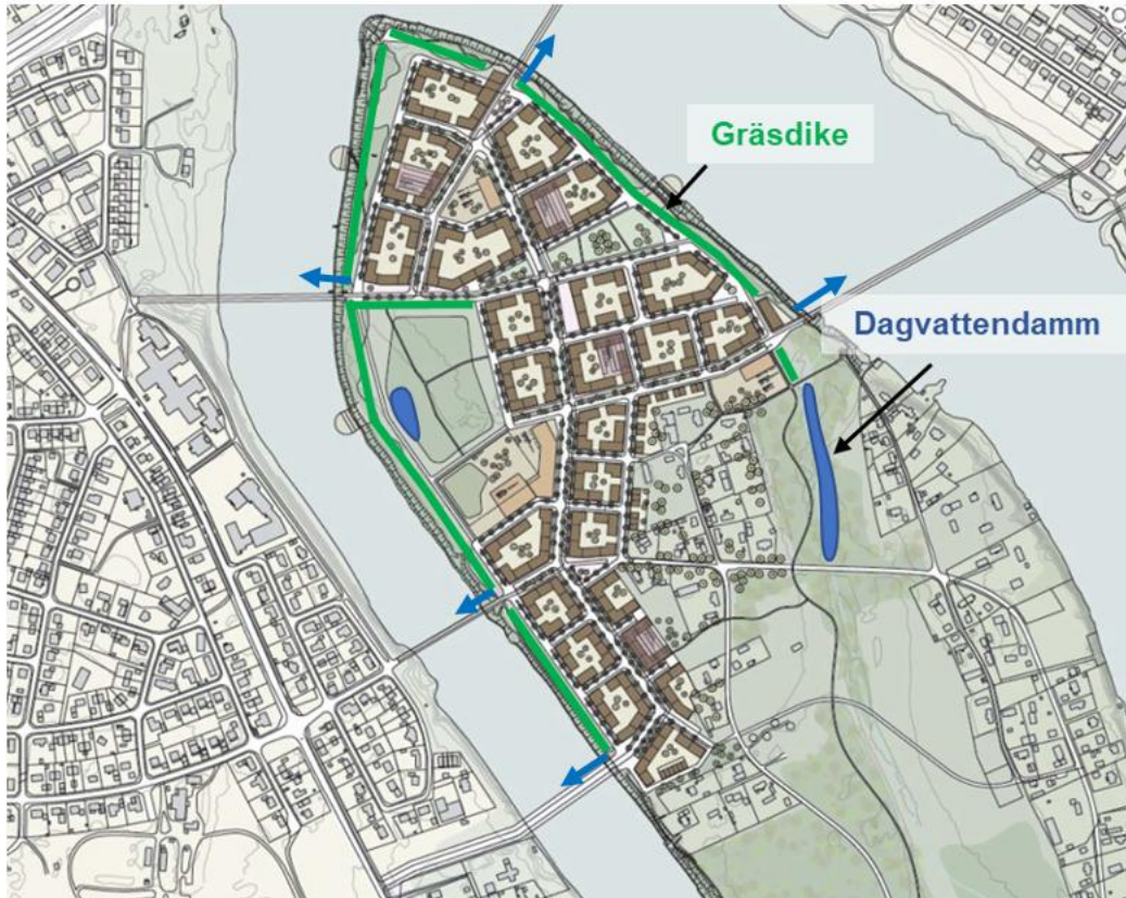
Figur 20. I figuren presenteras en systemlösning för planområdet som består av dagvattenledningar, gräsdiken och dagvattendamm.
