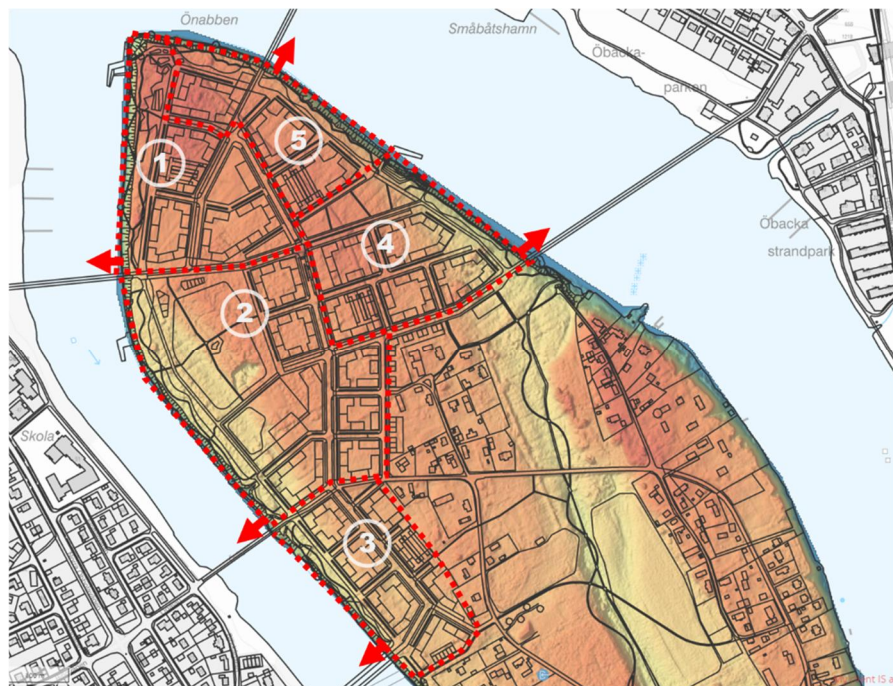
Figur 19. I figuren visas den indelning som tillämpats för avrinningsområden inom planområdet.
