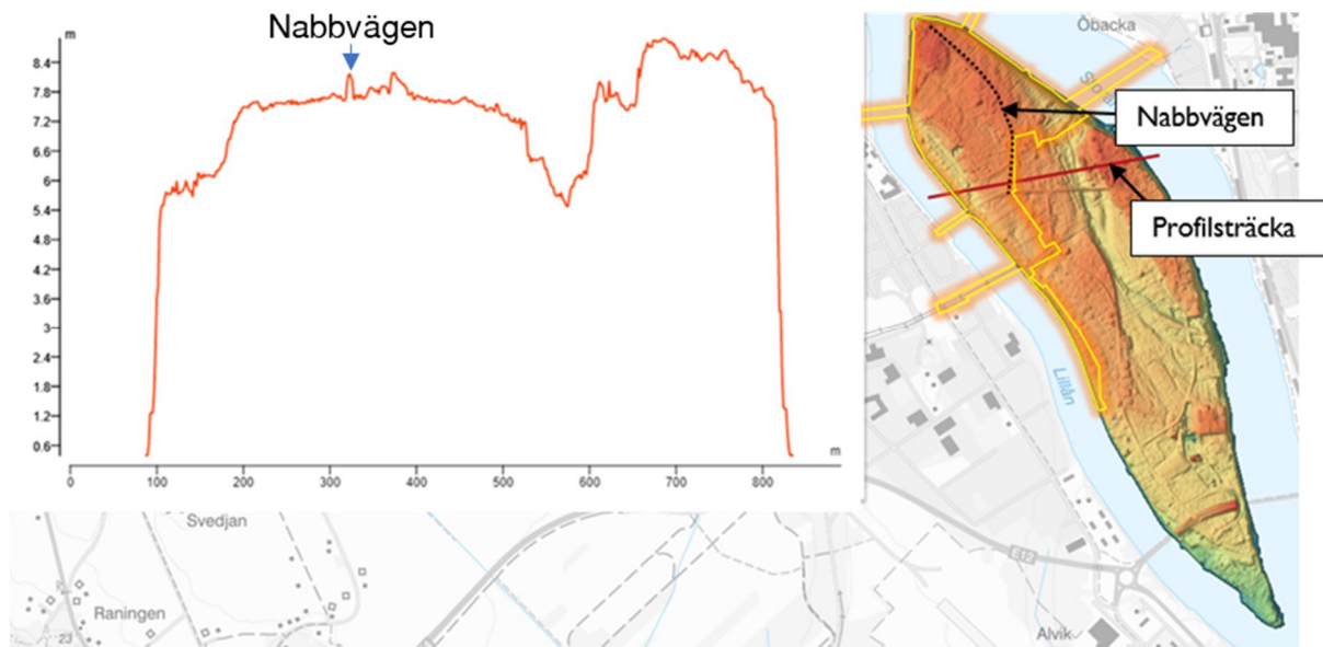
Figur 2. Terrängkarta över planområdet samt en profil dragen över planområdet (rött streck) för att illustrera hur branta älvbrinkarna är (ScalگوLive, 2020). Nabbvägen är markerad i svartstreckad linje och planområdet i gul linje.
