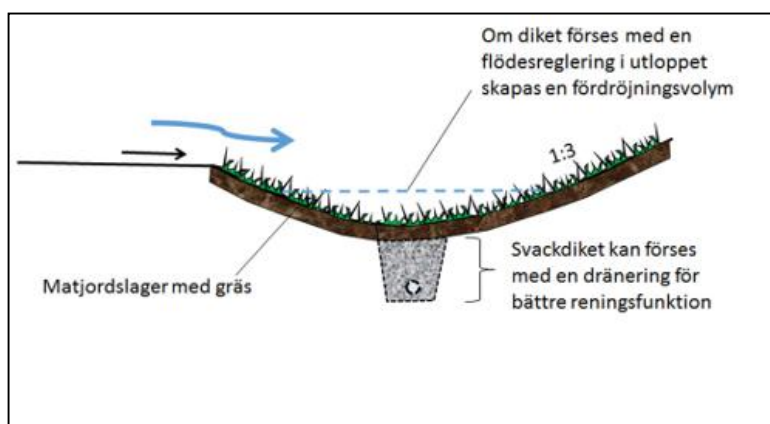
Figur 26. Principskiss samt exempelbild på ett gräsbeklätt svackdike (Bildkälla: WRS, 2017).
