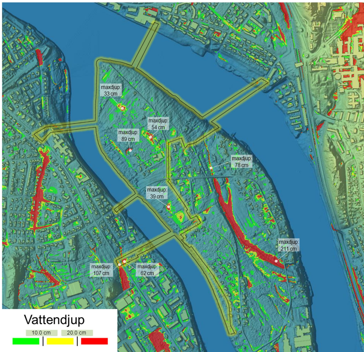
Figur 11. Översiktlig lågpunktskartering som visar vart det ansamlas vatten i dagsläget. Vattendjupet upp till 10 cm markerat med grön, från 10 cm upp till 20 cm är gul, från 20 cm och djupare är rött samt maxdjupet för några lågpunkter redovisas (ScalcoLive, 2020).
