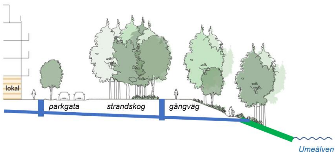
Figur 21. Avledning med dagvattenledningar i kombination med ett erosionsskyddat dike med utlopp i älven.
