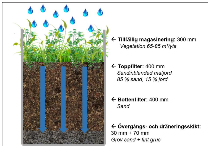
Figur 28. En principskiss för hur en nedsänkt växtbädd kan utformas (WSP, 2019).
