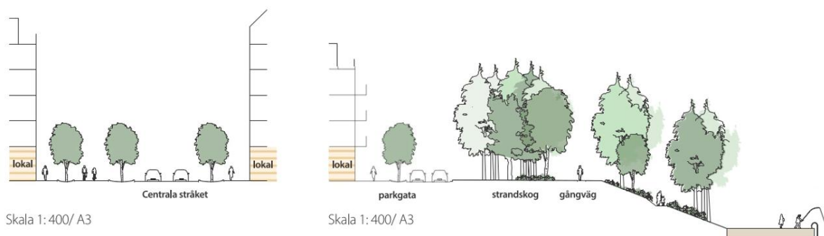
Figur 18. Sektioner för hur gator och strandpromenaden kan utformas inom planområdet enligt kvalitetsprogrammet (Umeå kommun, 2020).
