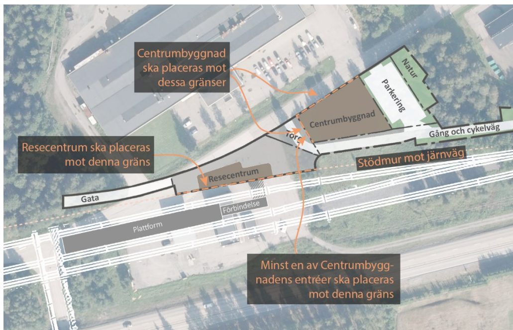
Figur 35. Illustration som redovisar planförslagets placerings- och utfromningsbestämmelser.
