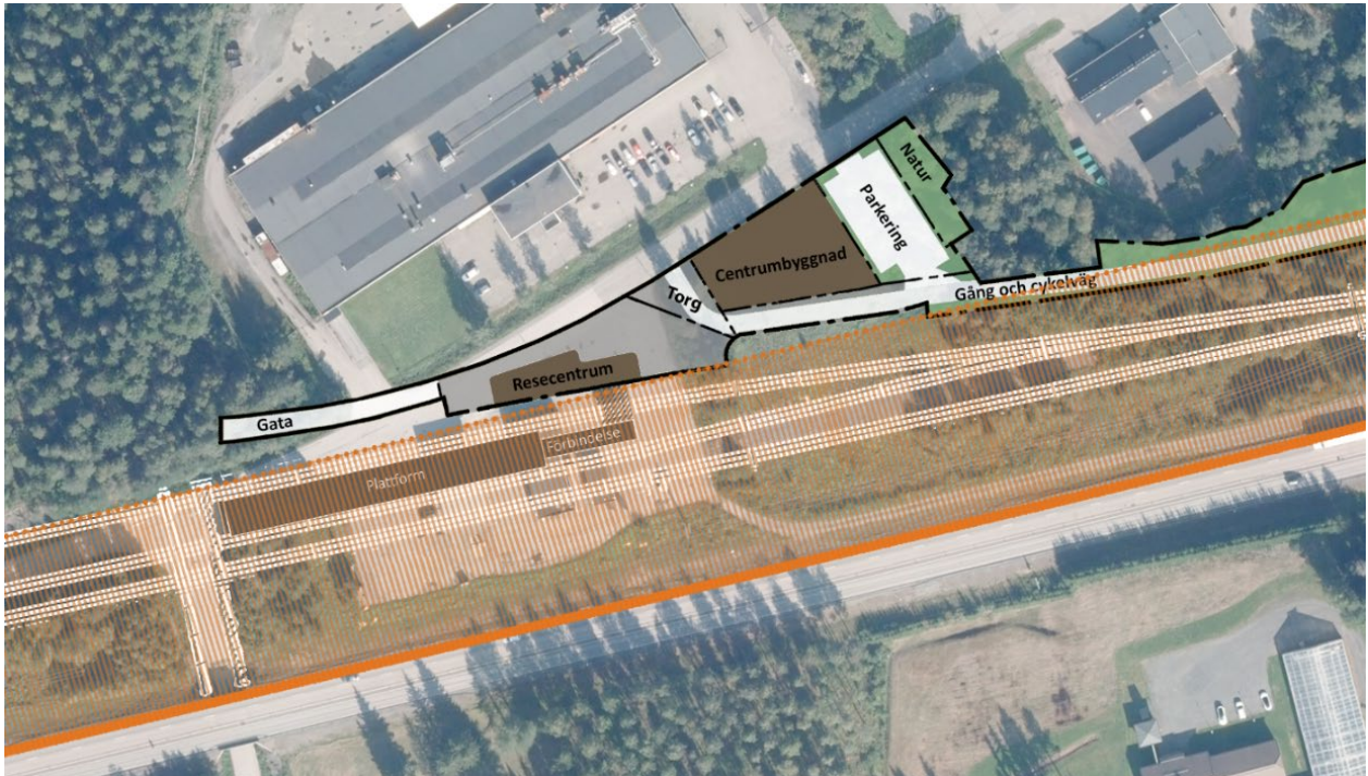
Figur 43. Illustration som redovisar en förstorad bild av stationsområdet för vägkant för E4:an är med orange heldragen linje. Illustrationen redovisar även ett 55 meter säkerhetsavstånd från vägen med prickad orange linje samt svag orange skraffering.
