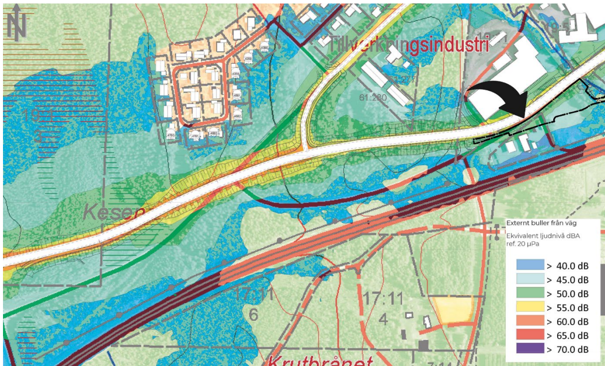
Figur 28. Ekvivalentbuller efter omdragning av Kungsvägen. Källa: WSP.
