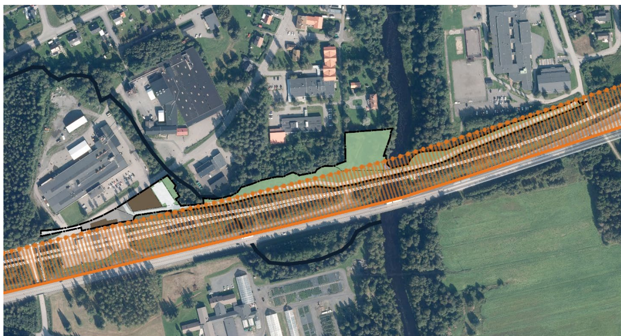
Figur 42. Illustration som redovisar vägkant för E4:an med orange heldragen linje. Illustrationen redovisar även ett 55 meter säkerhetsavstånd från vägen med prickad orange linje samt svag orange skraffering.
